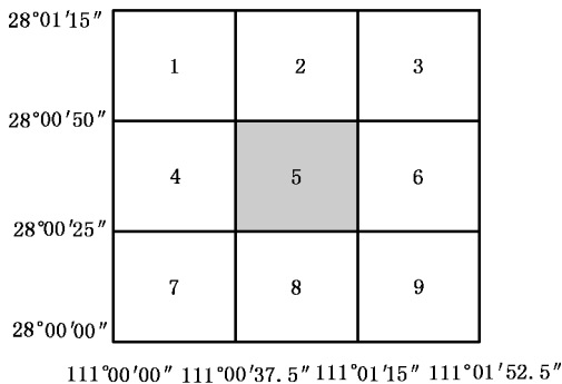
图 5 1 : 2 000 地形图的经、纬度分幅顺序编号
